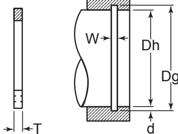
Groove Dimensions
